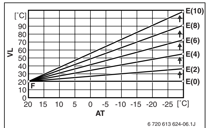
Sl. 25 Povečanje končne točke ogrevalne krivulje krogotoku mešalnega ventila
