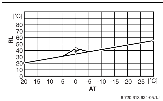
Sl. 24 Povečanje sobne temperature za 8 K (°C) pri temperaturni točki 0 °C
