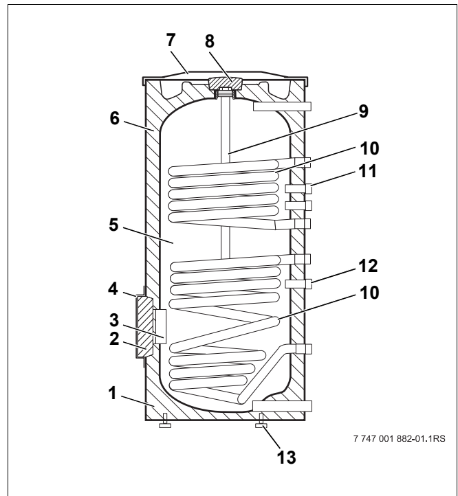
Sl. 1 Bojler SM300/1
