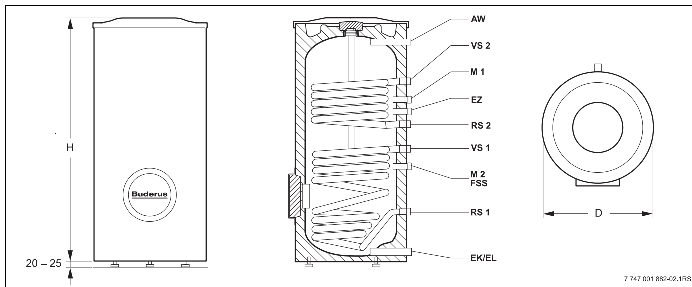
Sl. 2 Dimenzije in priključki (mere v mm)
